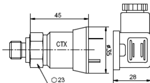
DIN 43650 connector
